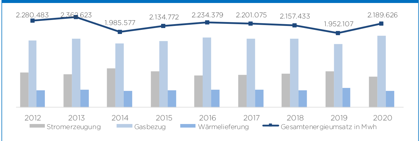
Abb. G1: Energiemix und Gesamtenergieumsatz in Mwh
