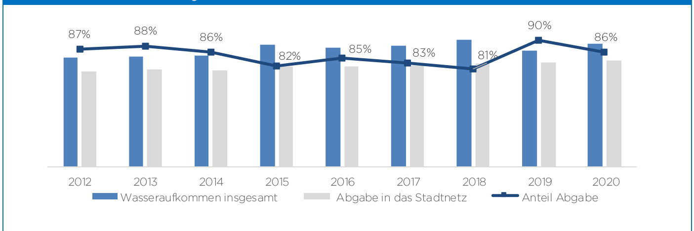
Abb. G2: Wasseraufkommen und Abgabe in das Stadtnetz
