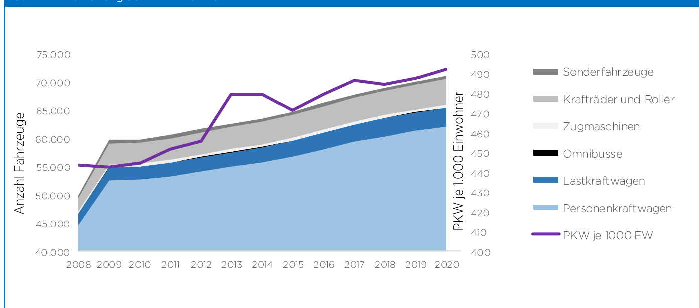
Abb. D4.1: Entwicklung der Kfz in Pforzheim
