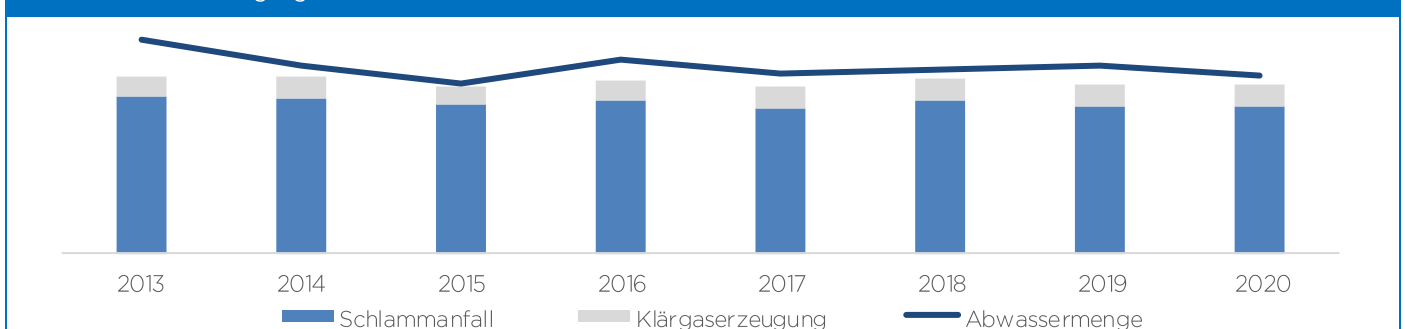
Abb. G4: Abwasserreinigung
